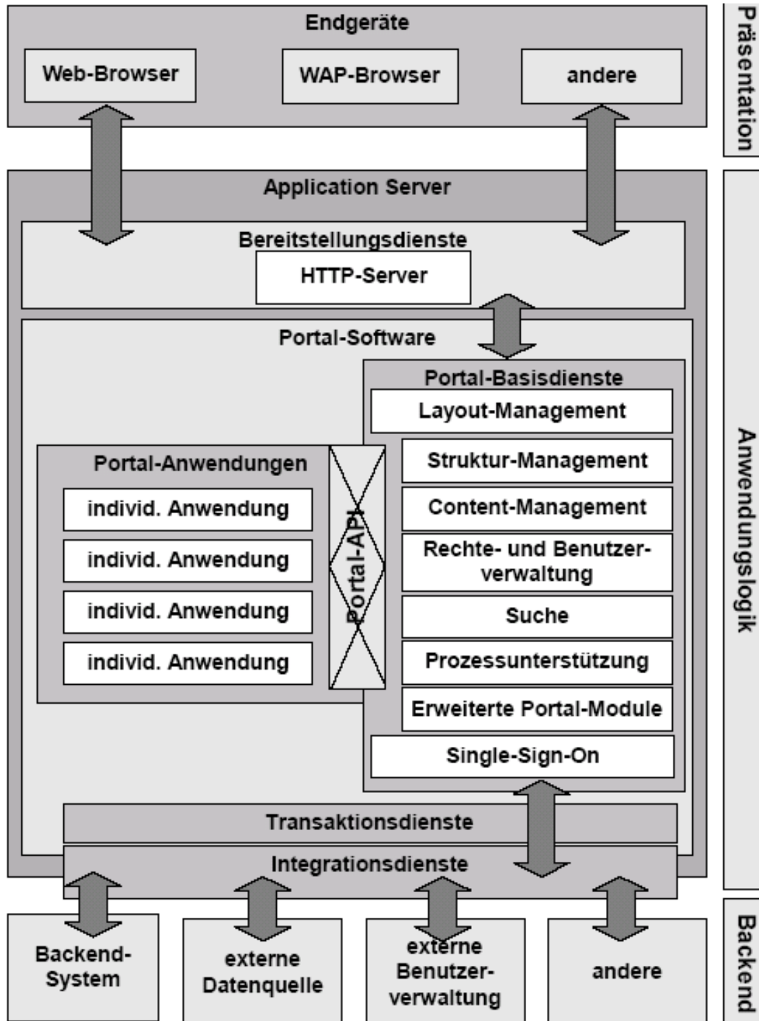
Referenzmodell für Portalsoftware (vgl. Kirchhof et al. 2004, S. 9).
